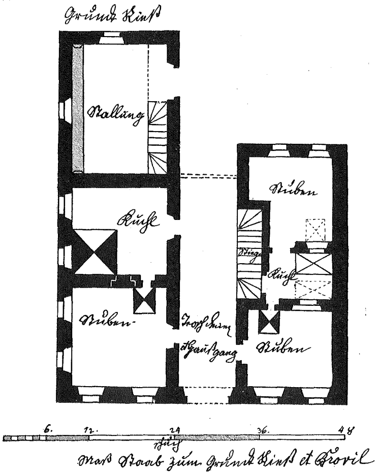
Fig. 40—41. Grundriß und Aufriß einer Söllbehausung in Wilten 1770.
