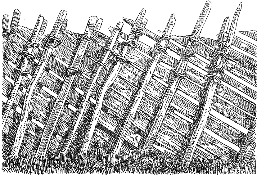
Fig. 24. Girscht'nzaun mit Wid'n.
