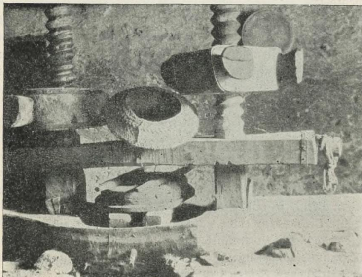
Abb. 12. Ölpreſse, Skutari.
