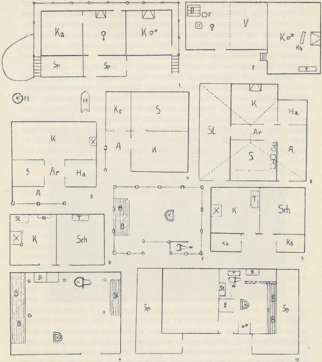
1. Haus, Singjonas bei Elbasan. Wohngeschoß. — 2. Haus, Vigu, Mirdita. — 3—5. Häuser der Muhadschir von Basar-Schjak bei Durazzo. — 6—8. Häuser der Aromunen, Durazzo. — 9. Haus der Aromunen, Hašmasej bei Pekinje. — 10—11. Häuser der Aromunen, Vila, Schkumbimündung.
